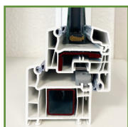
RENFORTS SELON ABAQUE, RENFORTS TOTAL EN OPTION
