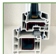
RENFORTS SELON ABAQUE, RENFORTS TOTAL EN OPTION
